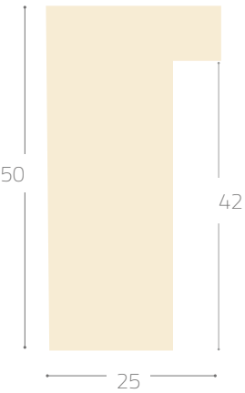
Profile 1184#
