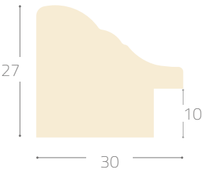
Profile 3736#
