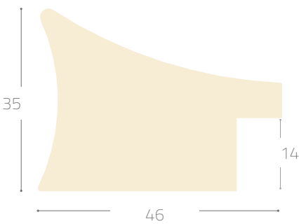
Profile 3044-C#
