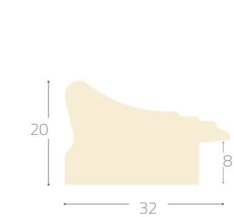
Profile 365#
