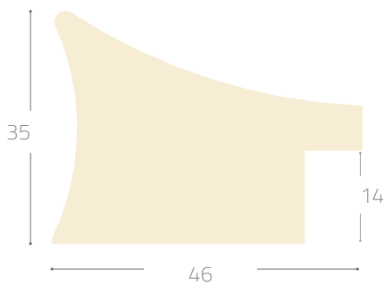
Profile 3044-C#
