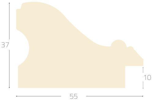
Profile 3014#
