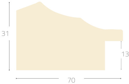
Profile 1215#
