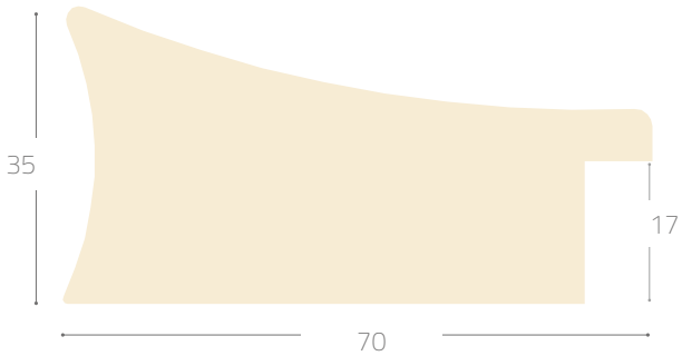
Profile 3043-C#
