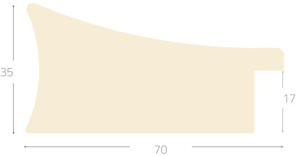
Profile 3043-C#
