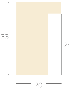
Profile 149#
